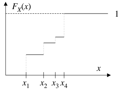
kertymäfunktio (kf)
