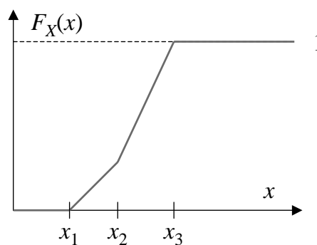
kertymäfunktio (kf)
