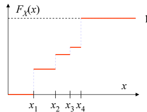
kertymäfunktio (kf)
