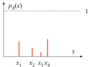
pistetodennäköisyysfunktio (ptnf)
